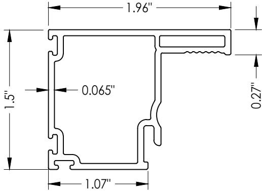
8 PLAIN STILE
